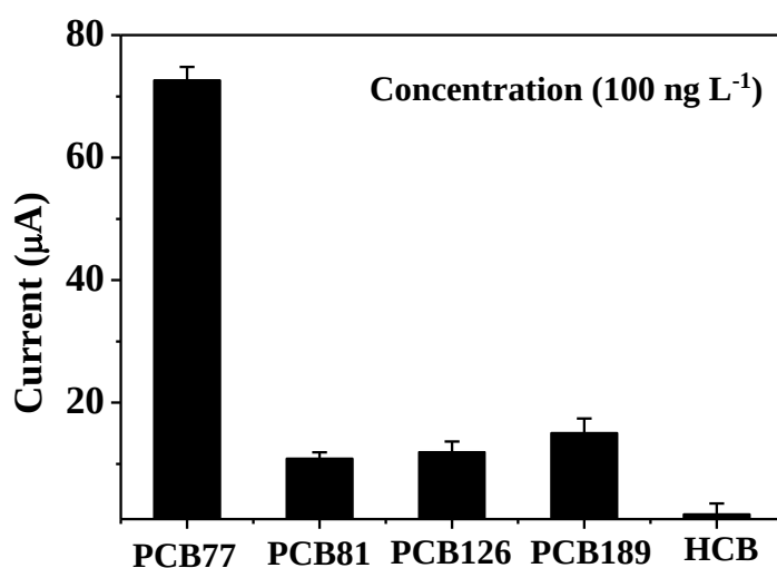
Fig 5. Screening of four PCBs (3,3',4,4'-PCB, PCB77; 3,4,4',5-PCB, PCB81; 3,3',4,4',5-PCB, PCB126; 2,3,3',4,4',5,5'-PCB, PCB189) and hexachlorobenzene (HCB) using the PP-AuNP-Ap/Au biosensor.
