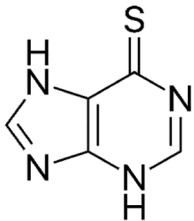
Mercaptopurine
