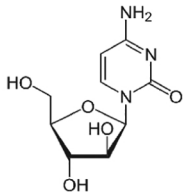
Cytarabine
