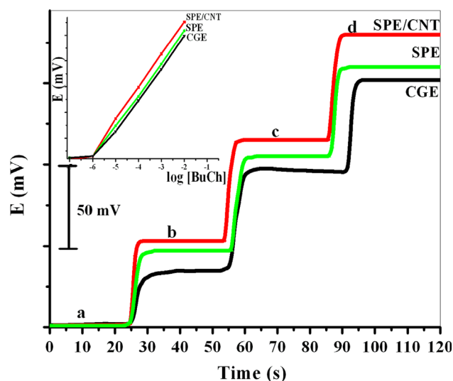
Fig. 1. Dynamic response of different BuCh sensors: (a) 1 \times 10^{-6} ; (b) 1 \times 10^{-5} ; (c) 1 \times 10^{-4} and (d) 1 \times 10^{-3} mol L ^{-1} BuCh solutions.
