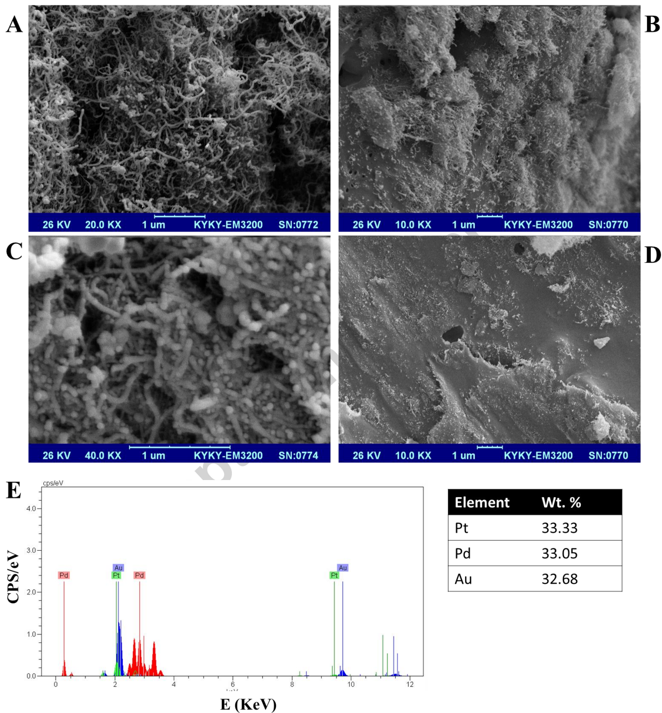
Fig. 3. The SEM image of (A) MWCNTs-IL/GCE, (B) Ch-IL/MWCNTs-IL/GCE, (C) PtAuPd NPs/Ch-IL/MWCNTs-IL/GCE and (D) HG-DDAB/PtAuPd NPs/Ch-IL/MWCNTs-IL/GCE. (D) Signature peaks obtained by EDS to characterize Pt, Au and Pd.
