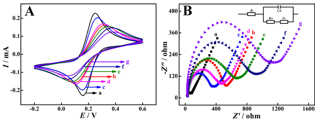
Figure 3. CV (A) and EIS (B) responses of (a) bare GCE, (b) GCE/CSZS-V Zn , (c) GCE/CSZS-V Zn /Au layer, (d) GCE/CSZS-V Zn /Au layer/H 2 , (e) GCE/CSZS-V Zn /Au layer/H 2 /HT, (f) GCE/CSZS-V Zn /Au layer/H 2 /HT/output DNA, and (g) GCE/CSZS-V Zn /Au layer/H 2 /HT/output DNA/H 3 -SiO 2 .
