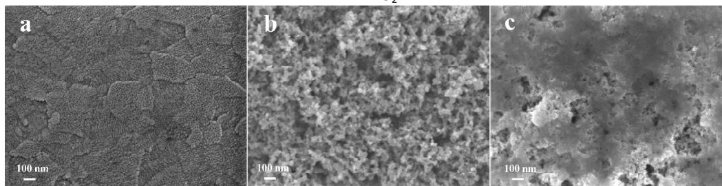
Fig. 1 SEM images of (a) bare ITO, (b) ITO/TiO 2 , (c) ITO/TiO 2 /CdS:Mn.
